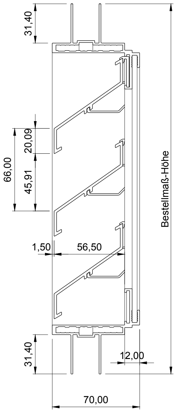
Vorderansicht
