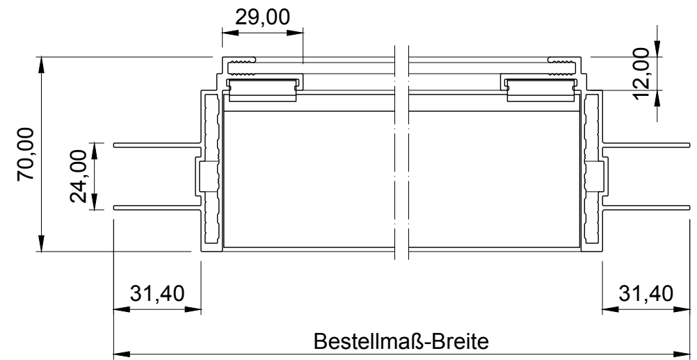
Draufsicht
