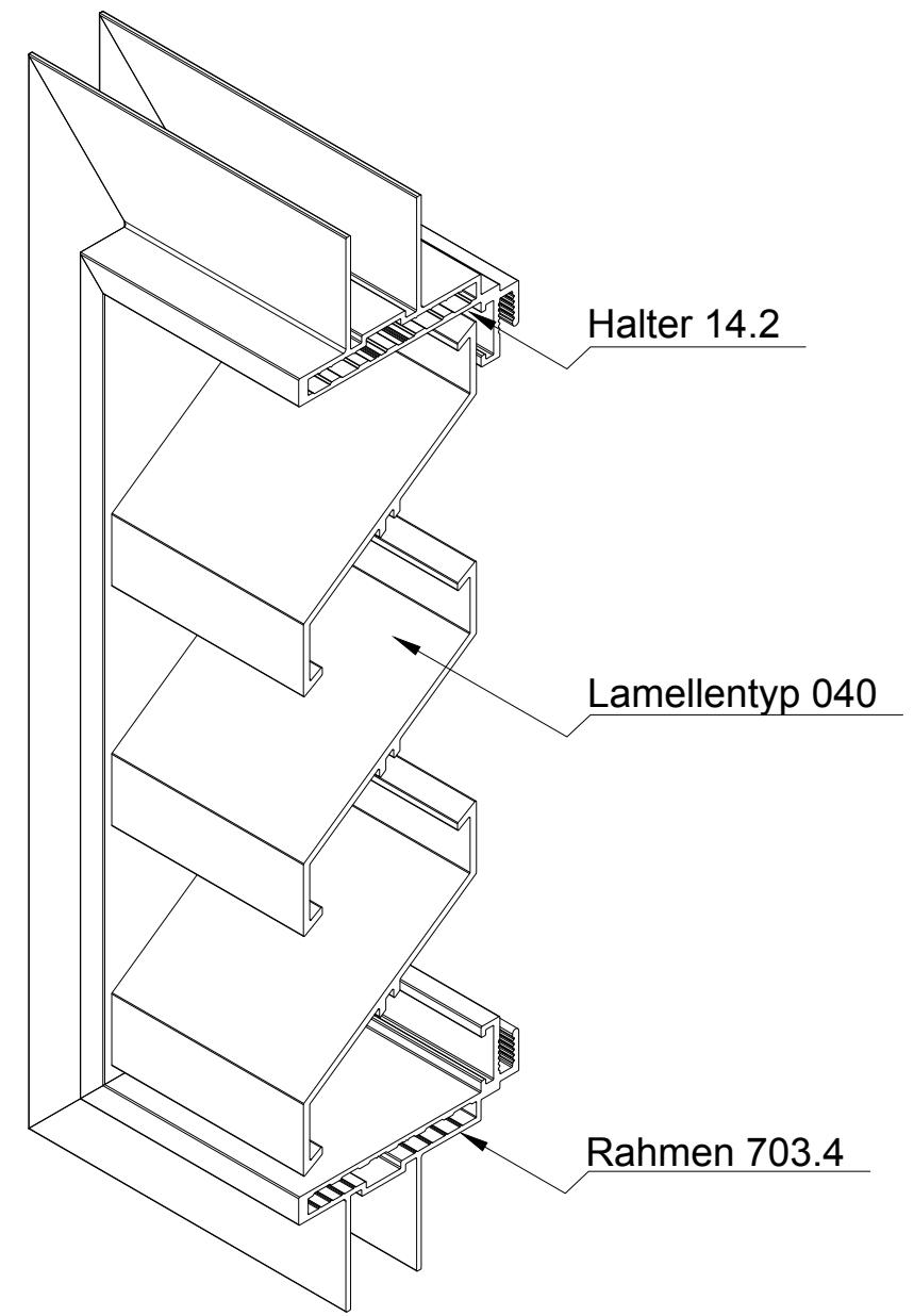
ISO-Ansicht
