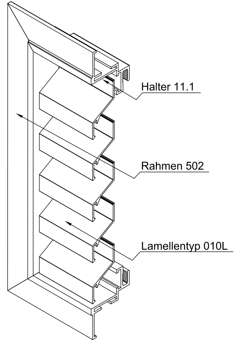
ISO-Ansicht
