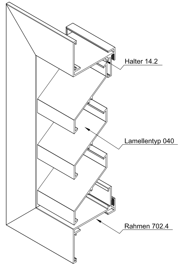
ISO-Ansicht
