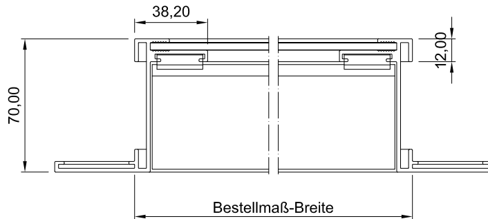
Draufsicht
