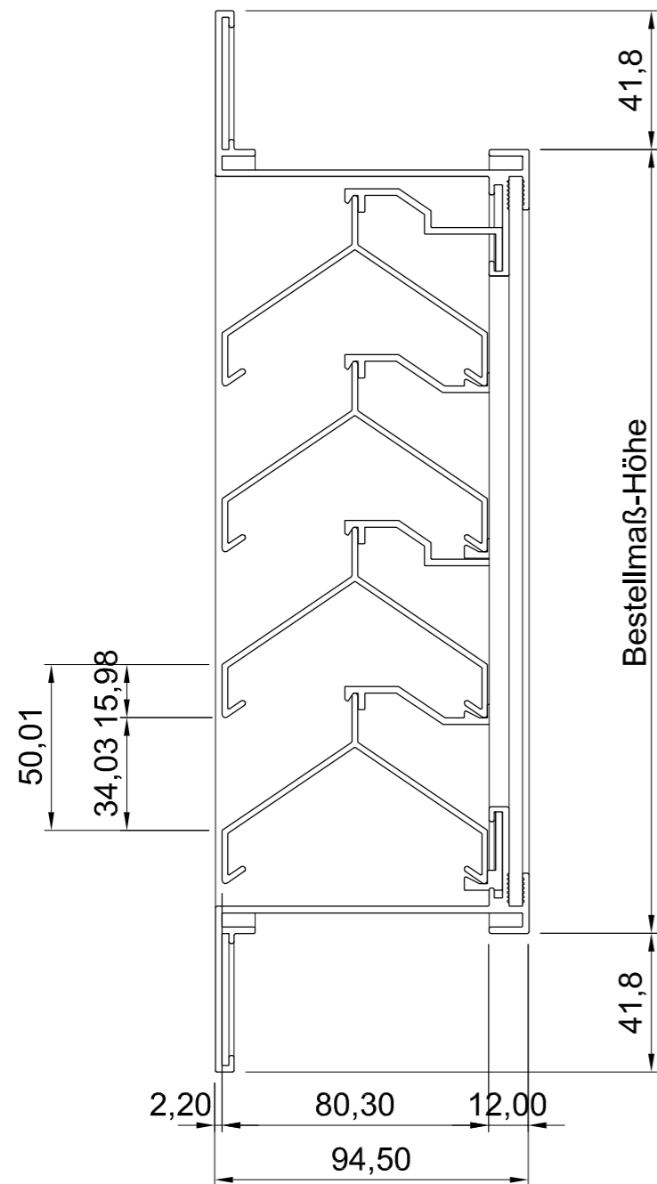
Vorderansicht
