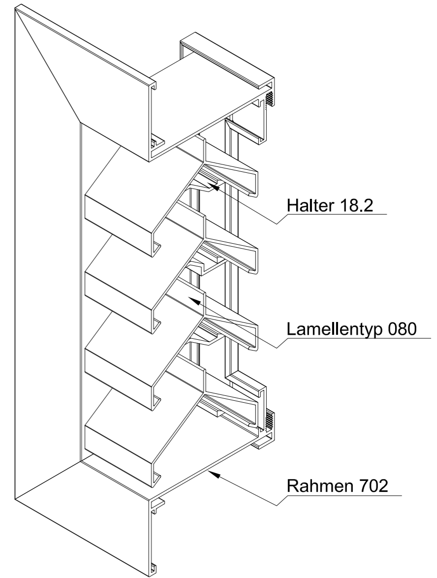
ISO-Ansicht
