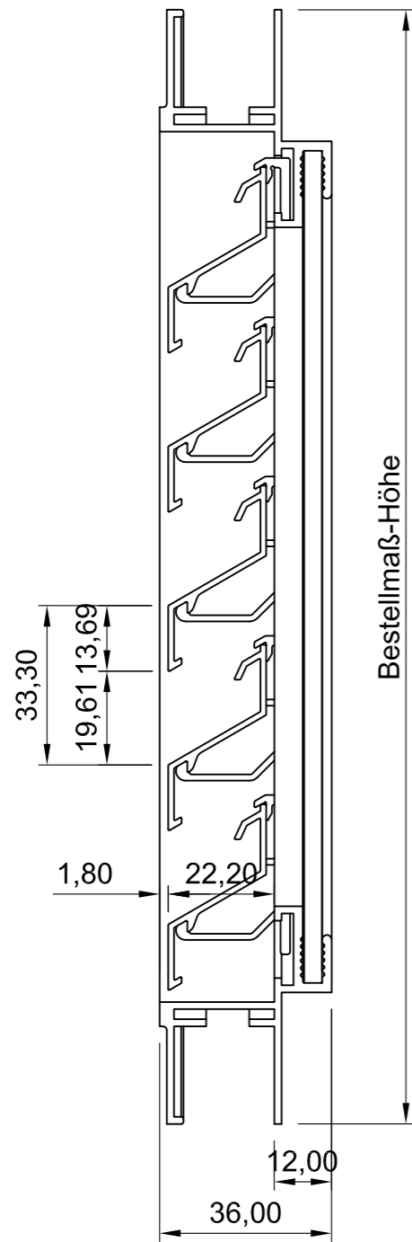
Draufsicht
