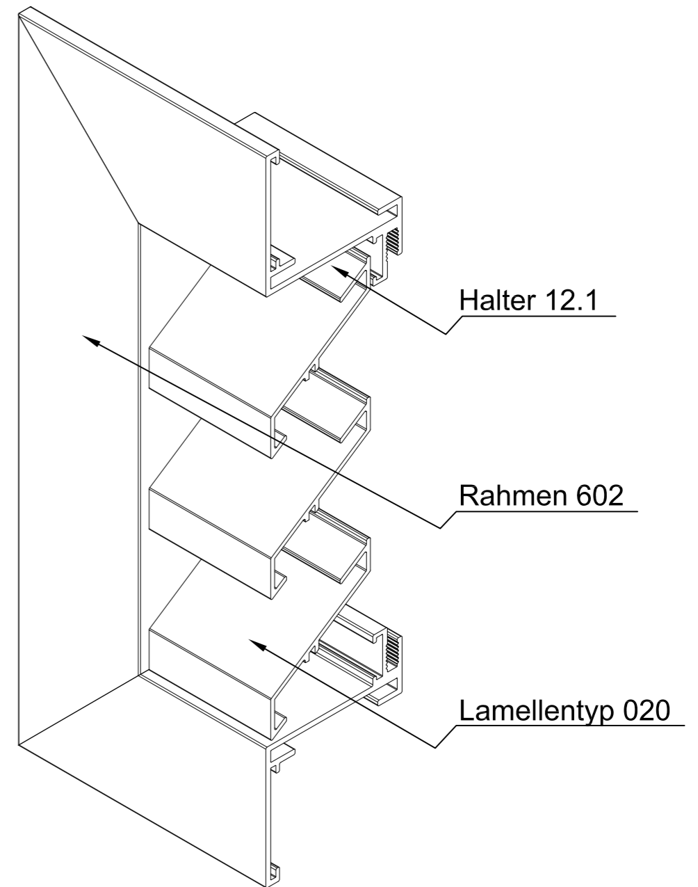
ISO-Ansicht
