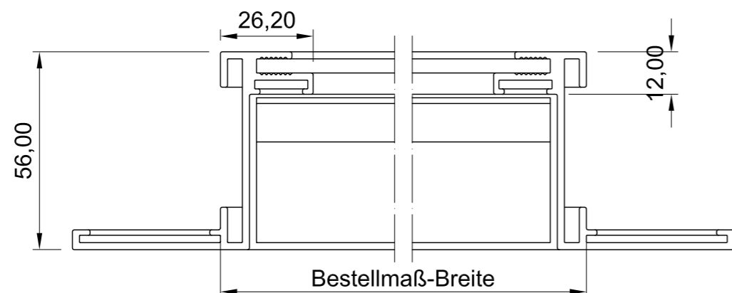
Draufsicht
