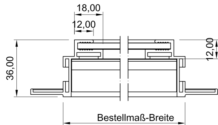
Draufsicht
