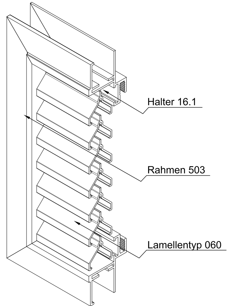
ISO-Ansicht
