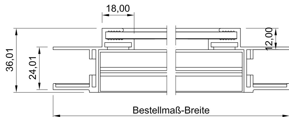
Draufsicht
