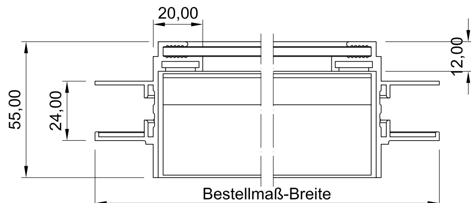
Draufsicht
